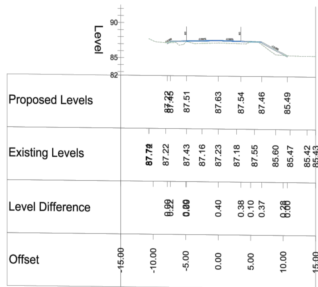
Chainage 700.000
